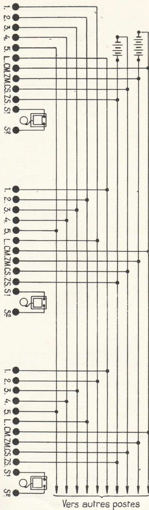
N° 560. — Schéma d'installation de Postes N° 300 ou 301 entre eux (Montage simple fil à Batterie Centrale)
