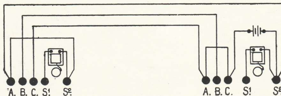
N° 57 ter. — Schéma d'installation de 2 Postes N° 400 ou 402 à appel réciproque (Montage primaire à 3 fils)
