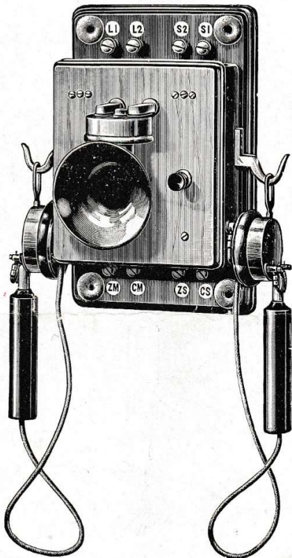
Poste Téléphonique Mural, type N° 1
